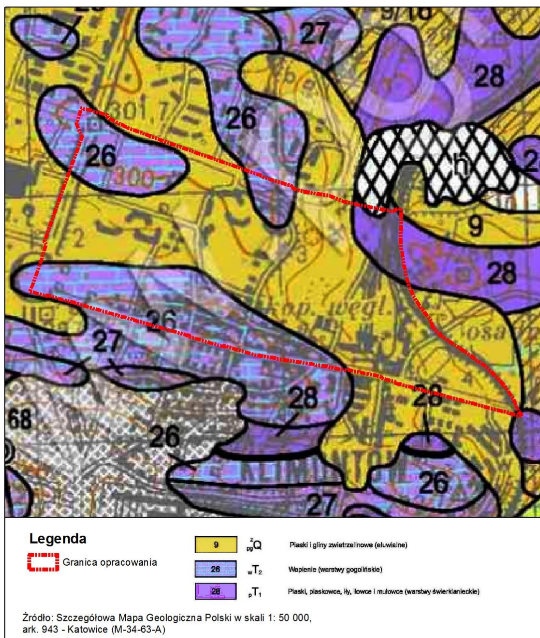
Rys. 2. Poglądowa budowa geologiczna terenu opracowania
